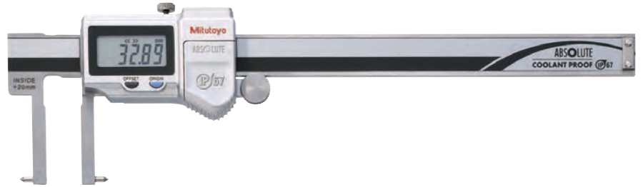
573-646 Hegyes mérőcsőr
