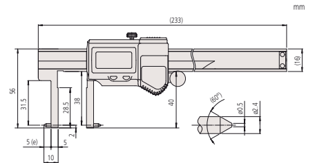
Hegyes mérőpofával
