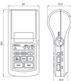
Méreték mm-ben
