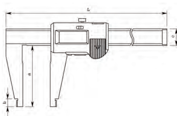
Mérőpofa kerekített felülettel belső mérésekhez
